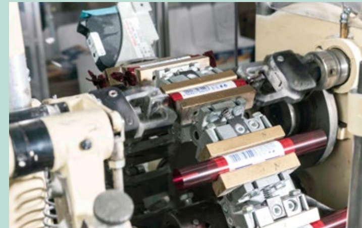
Rollenpackmaschine
